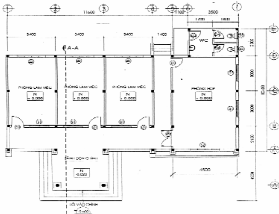
MẶT BẰNG NHÀ VĂN PHÒNG TL 1 / 100
