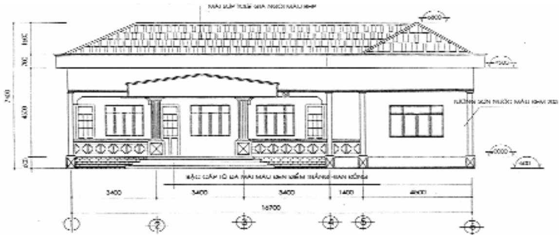
MẶT ĐỨNG CHÍNH NHÀ VĂN PHÒNG TL 1 / 100
